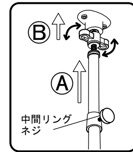
部品図 【突っ張りパイプ伸縮の注意】参照
